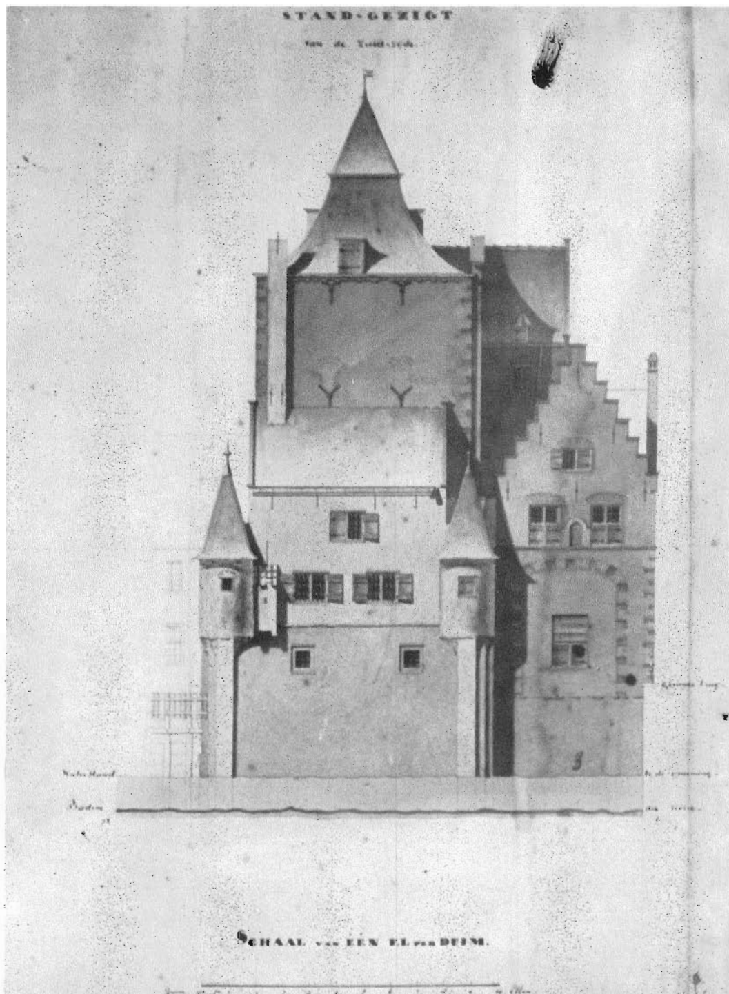
14. De Gevangentoren op de hoek Molenstraat/Oude Vest in 1828. Opmetingstekening door de stadsarchitect Koelewijn de Geus. Afgebroken in 1828. Foto Th. van Groesen. Stedelijk Museum, Breda.
